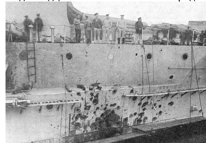
Повреждения броневых пояса «Евстафия»
