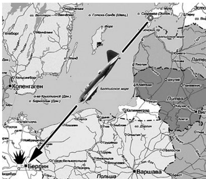
Схема первого авианалёта на Берлин 8 августа 1941 г.
